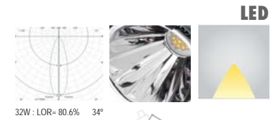
32W : LOR= 80.6% 34°
