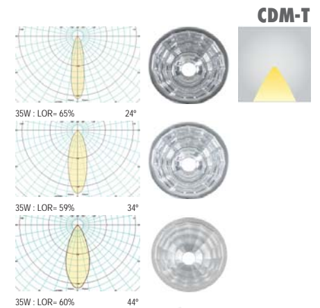
35W : LOR= 60% 44°
